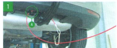
Fädeln Sie den Federhaken durch die Sicherungsöse (A) / Langlochbohrung an der Anhängerkupplungstraverse und formen Sie zusätzlich die Schlaufe um den Kugelhals; Klinken Sie den Haken am Seil ein.
